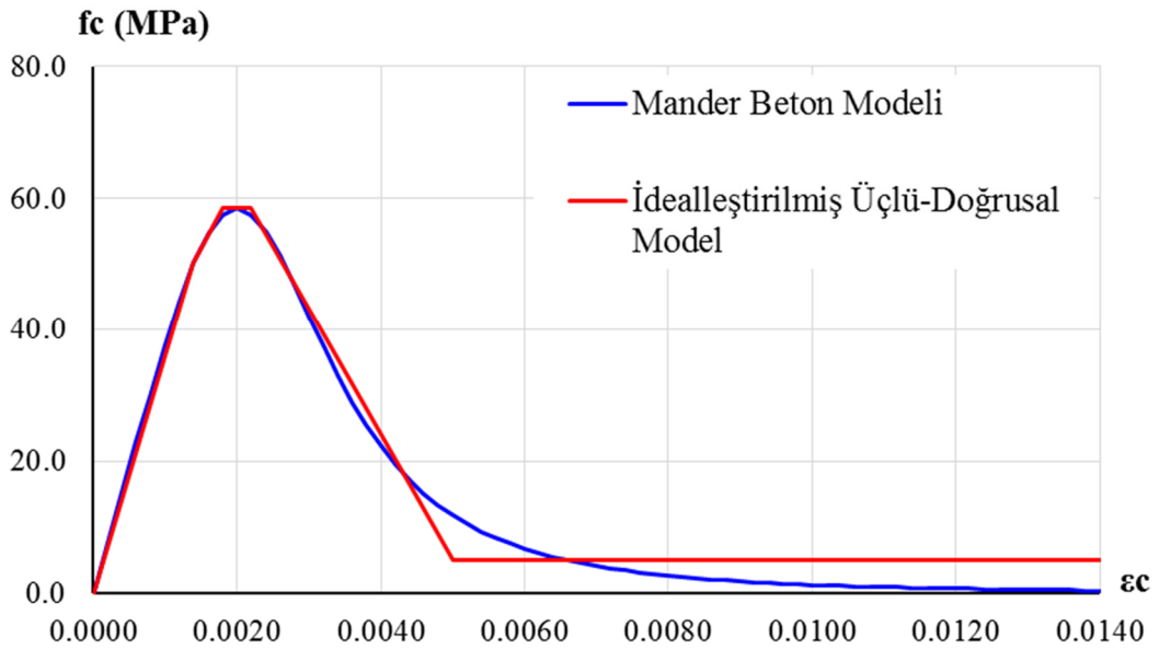
Şekil 5.5 Sargılanmamış beton modeli
