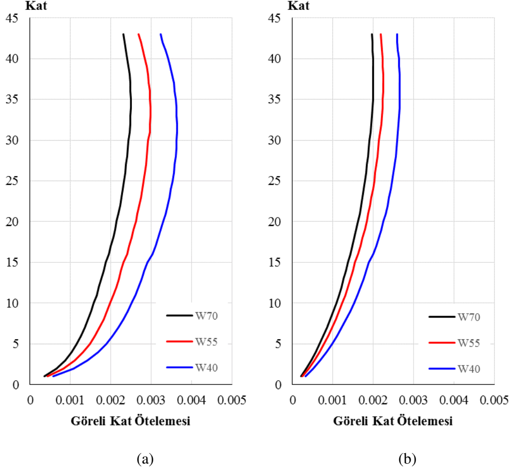
Şekil 4.13 (a) X doğrultusu göreli kat ötelemeleri (b) Y doğrultusu göreli kat ötelemeleri
