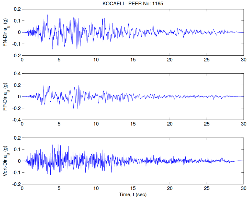
Şekil 5.19 Örnek bir deprem kaydı
