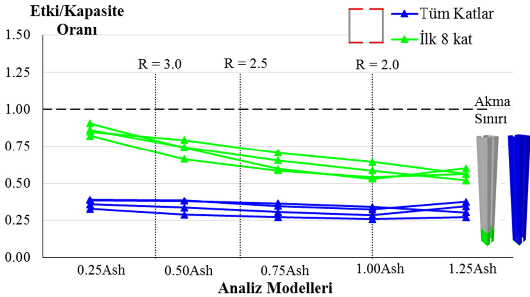
Şekil 5.36 6.5 m uzunluğundaki duvarlarda etki-kapasite oranları
