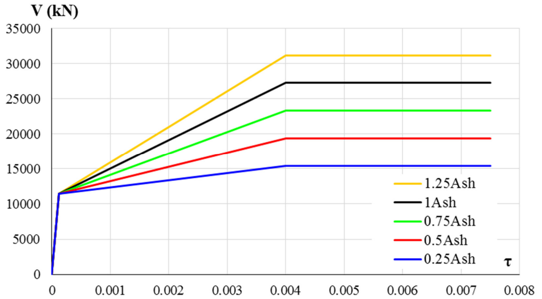
Şekil 5.18 Kontrol modellerinde 16 m uzunluğundaki duvar için örnek elastik ötesi kesme modelleri
