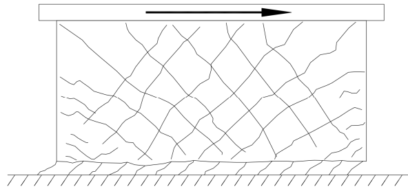
Şekil 2.6 Betonarme duvarlarda kayma güç tükenmesi(Paulay, Priestley ve Synge, 1979)
