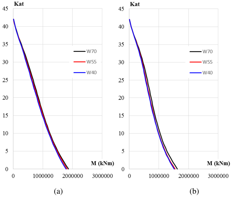
Şekil 4.12 (a) Y ekseninde devrilme momentleri (b) X ekseninde devrilme momentleri
