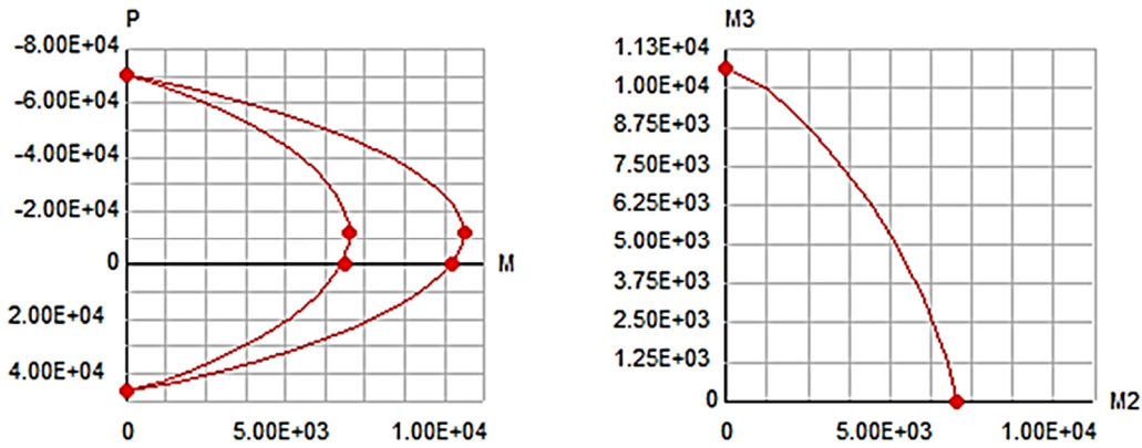
Şekil 5.4 Kompozit kiriş P-M-M mafsal özellikleri
