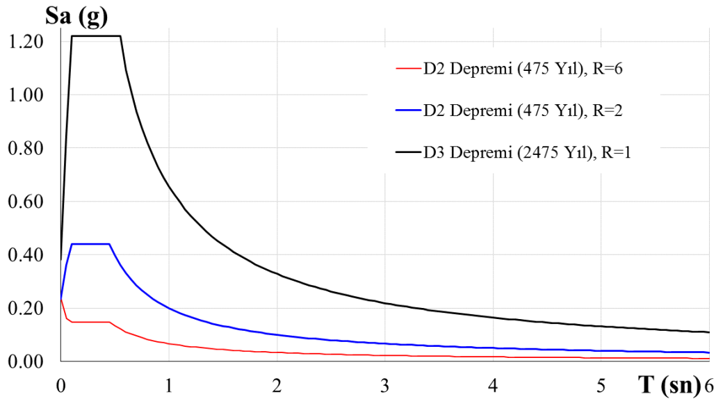
Şekil 3.4 Kullanılan ivme spektrumları
