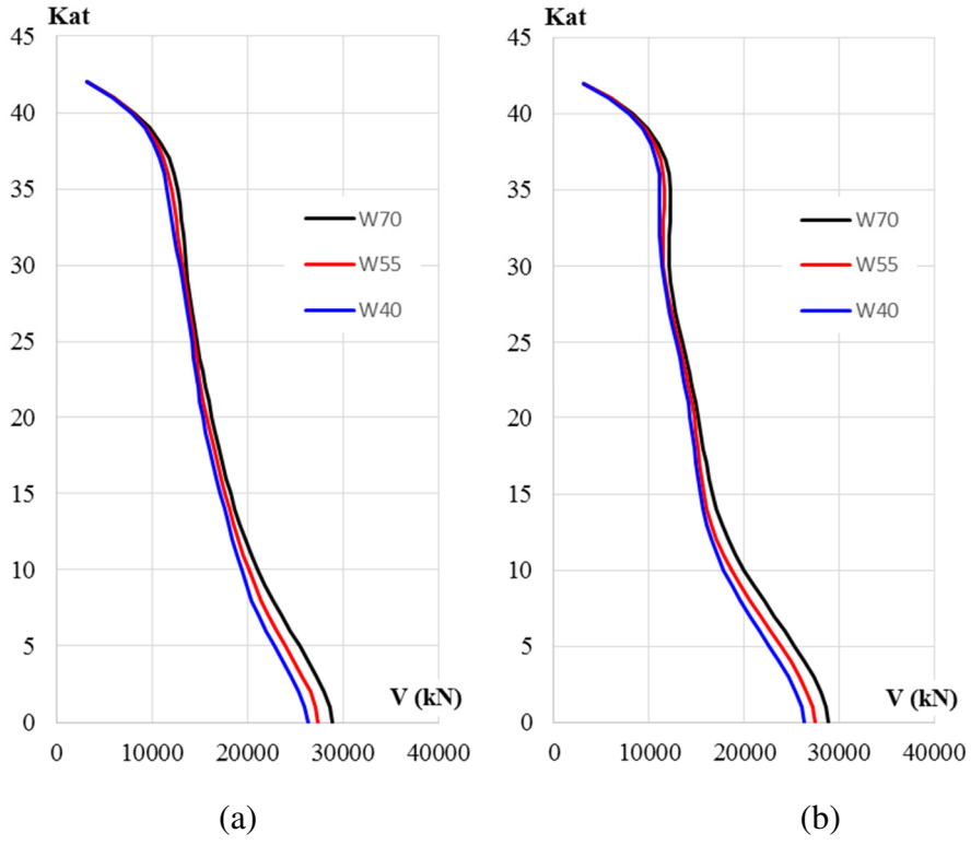
Şekil 4.11 (a) X doğrultusu kat kesme kuvvetleri (b) Y doğrultusu kat kesme kuvvetleri
