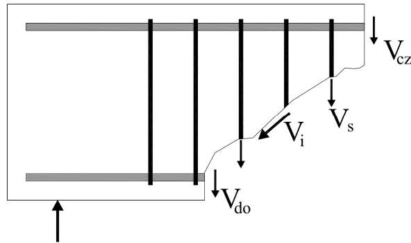
Şekil 2.1 Betonarme kesitte kesme direnci(Nilson, Darwin ve Nolan, 2009)
